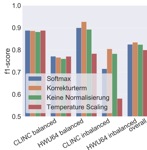
Abbildung 4 – Performance der unterschiedlichen Normalisierungsfunktionen.
