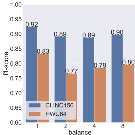
Abbildung 3 – Ergebnisse der Experimente mit inbalancierten DS.
