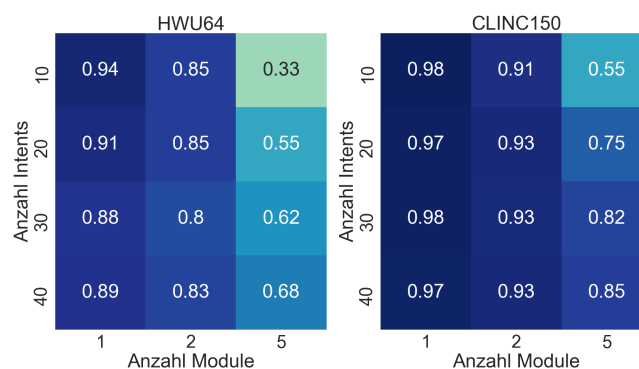
Abbildung 2 – F1-Scores abhängig von der Zahl der Intents insgesamt und der Zahl der Module im DS für beide Datasets im Experiment mit balancierten Modulen.
