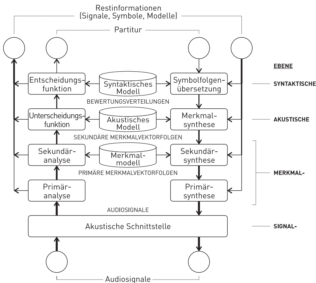
Bild 7 - Intelligentes System zur (akustischen) Signalverarbeitung [21].
