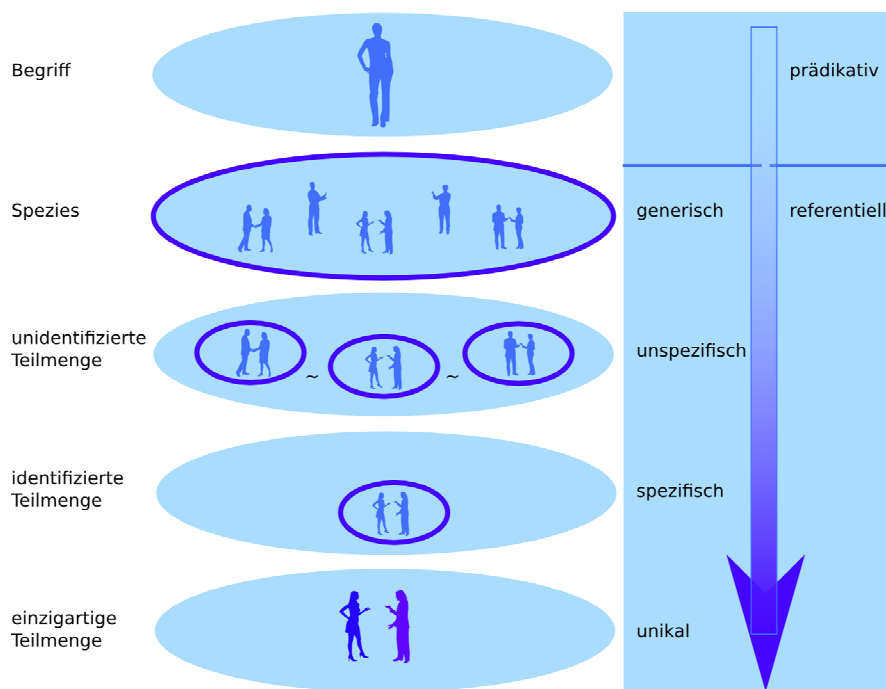
Abbildung 8 Schrittweise Individuation
