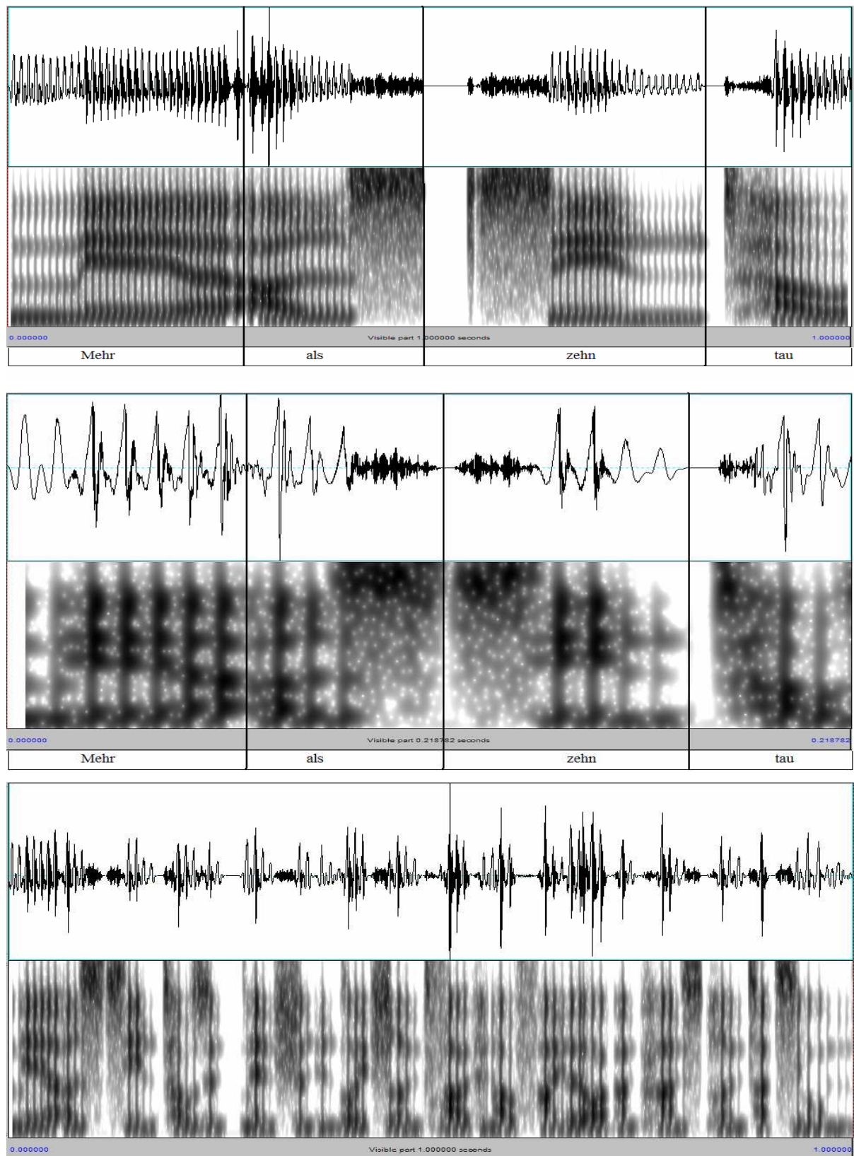
Abbildung 2 – Wellenform und Spektrogramm des Satzanfangs "Mehr als zehn tau(send ...)". Oben: 1,000 sek im Normaltempo (ca. 5 s/s). Mitte: 0,219 sek im Tempo 22 s/s. Unten: 1,000 sek im Tempo 22 s/s.
